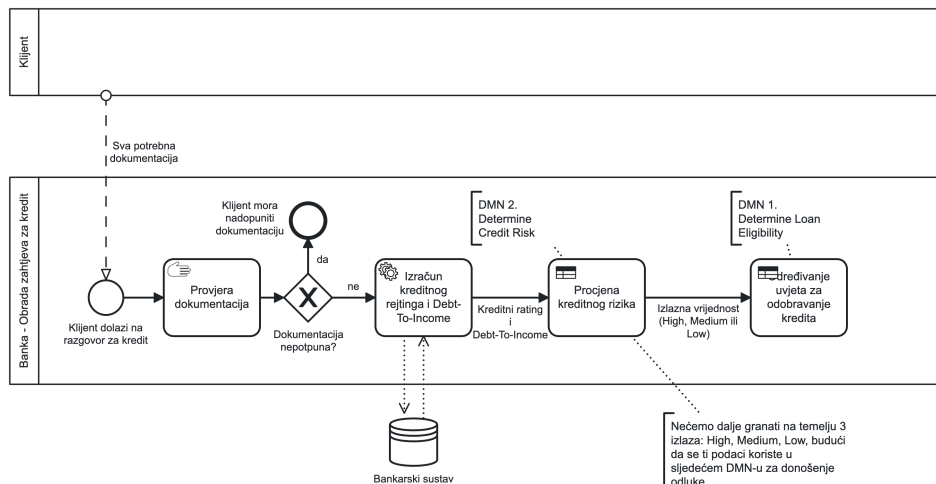
Slika 20. BPMN model: Određivanje uvjeta za odobravanje kredita koristeći DMN1 i DMN2 tablice odluka i Business Rule Task aktivnosti
