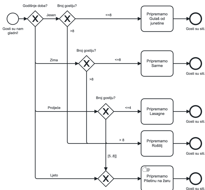
Slika 9. BPMN model: Priprema hrane na temelju godišnjeg doba i broja gostiju koristeći XOR skretnice (s dodatnim uvjetom za "Roštilj")
