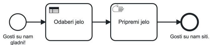
Slika 11. BPMN model: Priprema hrane na temelju DMN tablice odluke koristeći Business Rule Task za odabir jela (generalizirana verzija)
